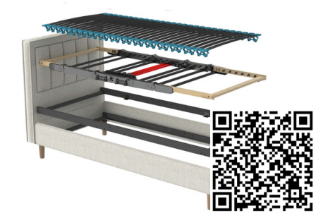
OCTO Motorlu Baza Mekanizması Motorized Bed Base Mechanism
